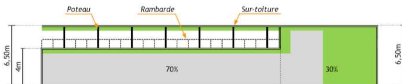
Cas d'une construction Bepos avec une toiture-terrasse accessible et sur-toiture
